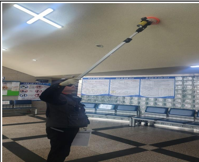
사진 설명 : 화재감지기 점검
